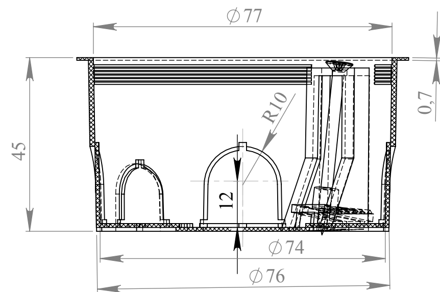
СЕЧЕНИЕ А-А
