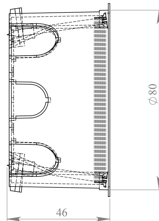
СЕЧЕНИЕ В-В
