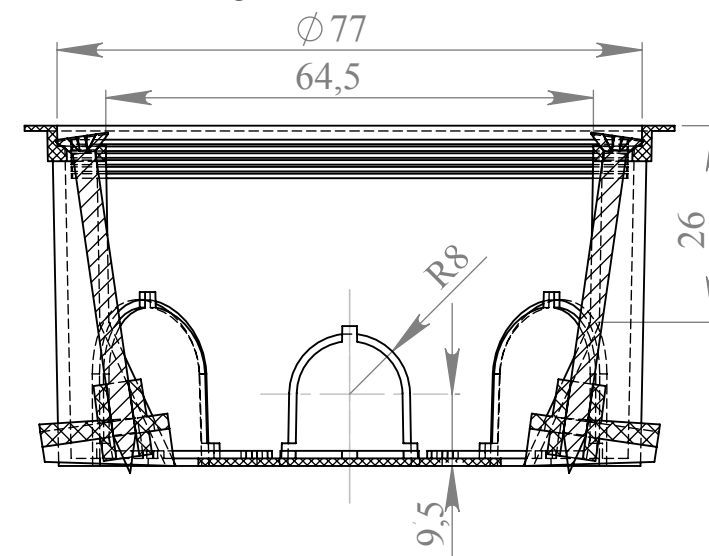
СЕЧЕНИЕ В-В
