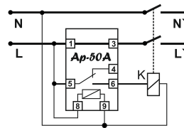
Схема подключения
